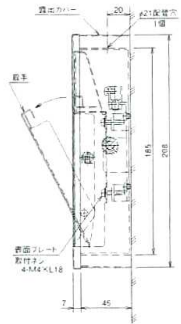
N-391A型( 型)
