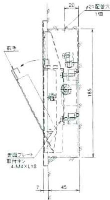
N-381A型(埋込型)
